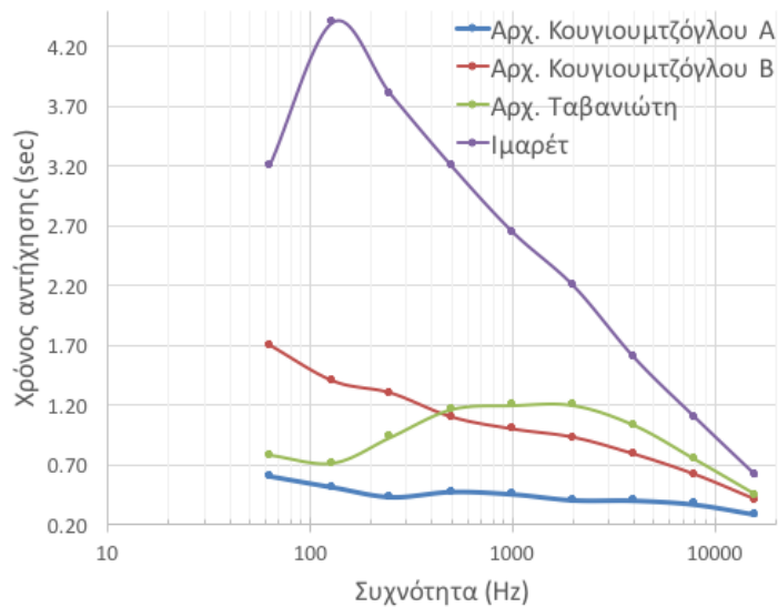
Σχήμα 1. Χρόνος αντήχησης χώρων εκδηλώσεων και μουσείων που μελετήθηκαν στα πλαίσια του παρόντος έργου συναρτήσει της συχνότητας.
