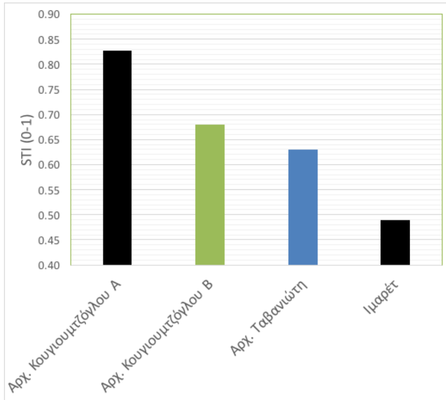
Σχήμα 3. Δείκτης μετάδοσης ομιλίας χώρων εκδηλώσεων και μουσείων που μελετήθηκαν στα πλαίσια του παρόντος έργου.
