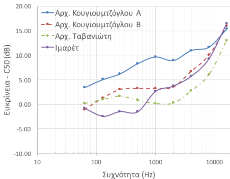
Σχήμα 2. Ακουστική ευκρίνεια (C50) για τους χώρους εκδηλώσεων και μουσείων που μελετήθηκαν στα πλαίσια του παρόντος έργου συναρτήσει της συχνότητας.
