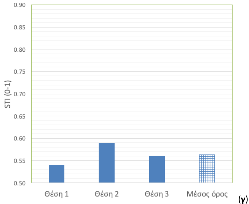
Σχήμα 3. Δείκτης Μετάδοσης Ομιλίας (STI) στο Γενί Τζαμί της Κομοτηνής. Η πηγή είναι τοποθετημένη στο μιχράμπ προσανατολισμένη προς (α) το Ιερό (Μέκκα), (β) προς τους πιστούς και (γ) τοποθετημένη στην εξέδρα (κιουρσού).
