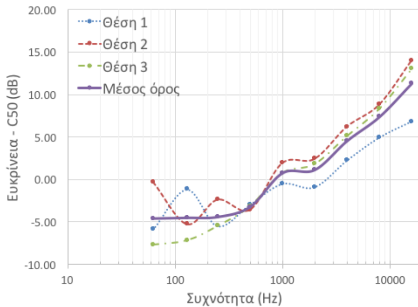
Σχήμα 2. Ακουστική ευκρίνεια (C50) συναρτήσει της συχνότητας στο Γενί Τζαμί της Κομοτηνής. Η πηγή είναι τοποθετημένη στο μικράμπ προσανατολισμένη προς (α) το Ιερό (Μέκκα), (β) προς τους πιστούς και (γ) τοποθετημένη στην εξέδρα (κιουρσού).
