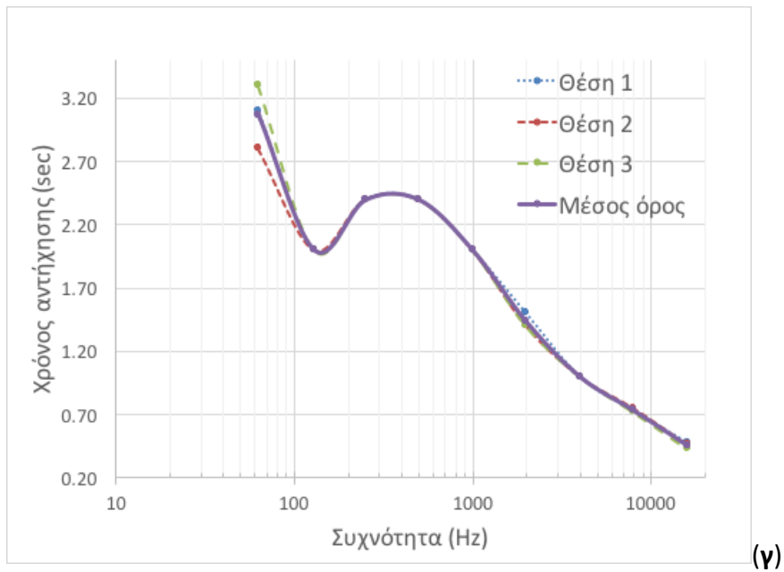
Σχήμα 1. Χρόνος αντίληψης συναρτήσει της συχνότητας στο Γενί Τζαμί της Κομοτηνής. Η πηγή είναι τοποθετημένη στο μικράμπ προσανατολισμένη προς (α) το Ιερό (Μέκκα), (β) προς τους πιστούς και (γ) τοποθετημένη στην εξέδρα (κιουρσού).
