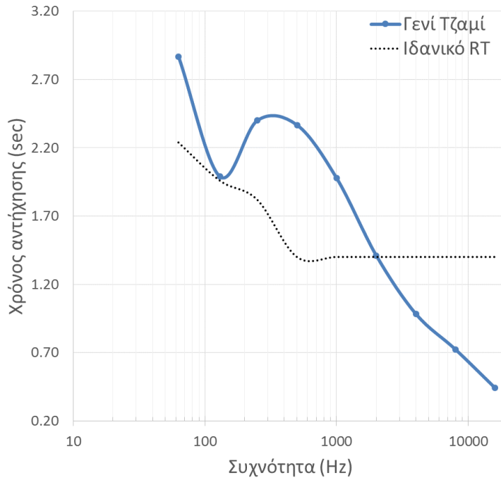
Σχήμα 4. Χρόνος αντήρησης συναρτήσει της συχνότητας στο Γενί Τζαμί της Κομοτηνής
